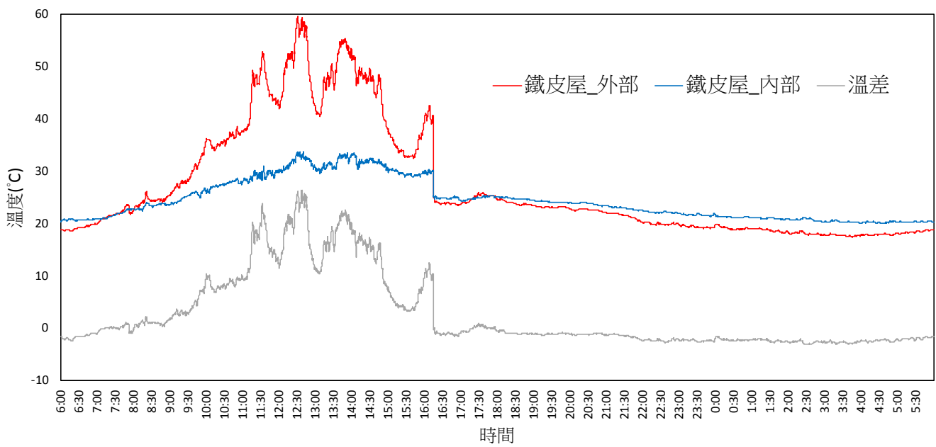
圖 10 真實環境中石板屋內外部溫度變化情形
