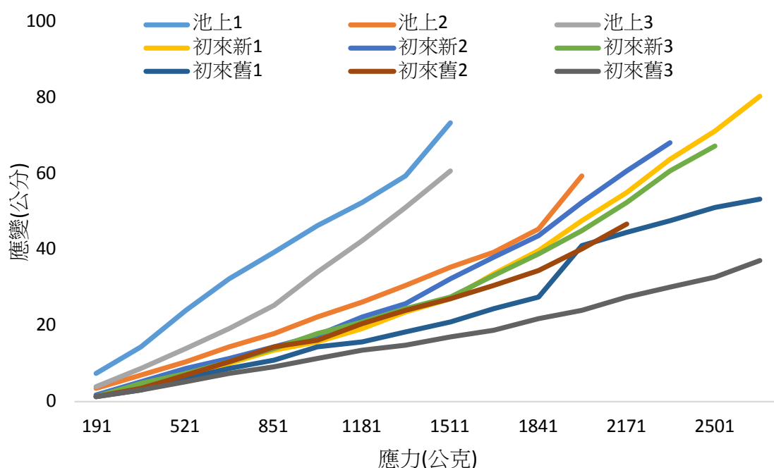
圖 7 竹子抗彎試驗結果
