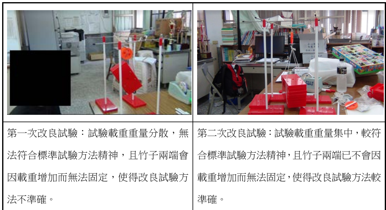
圖 3 竹子抗彎試驗過程
