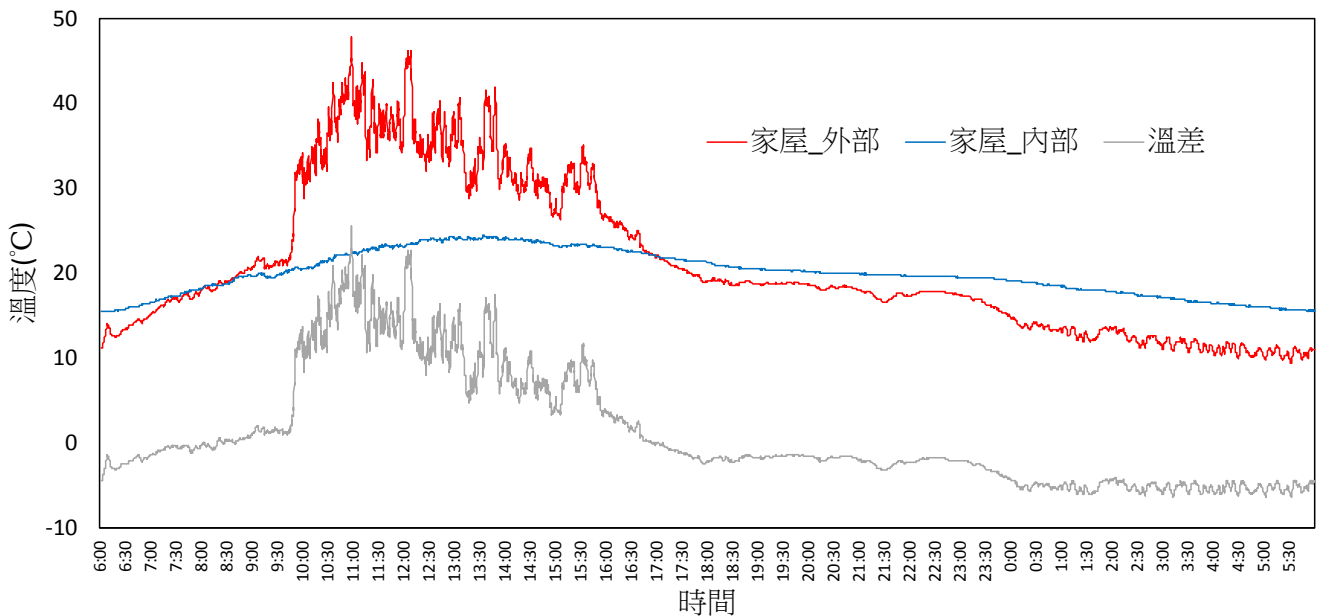
圖8 真實環境中竹屋內外部溫度變化情形
