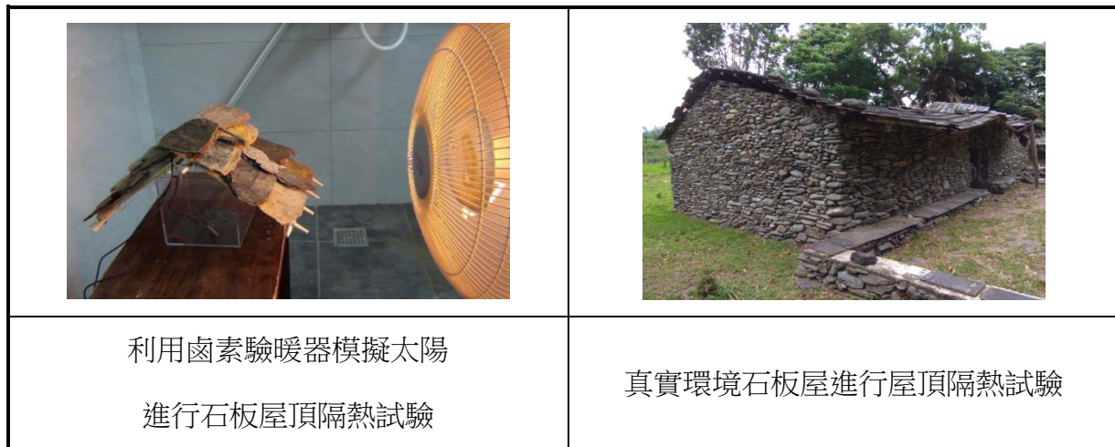
圖 6 外殼隔熱試驗試驗情形
