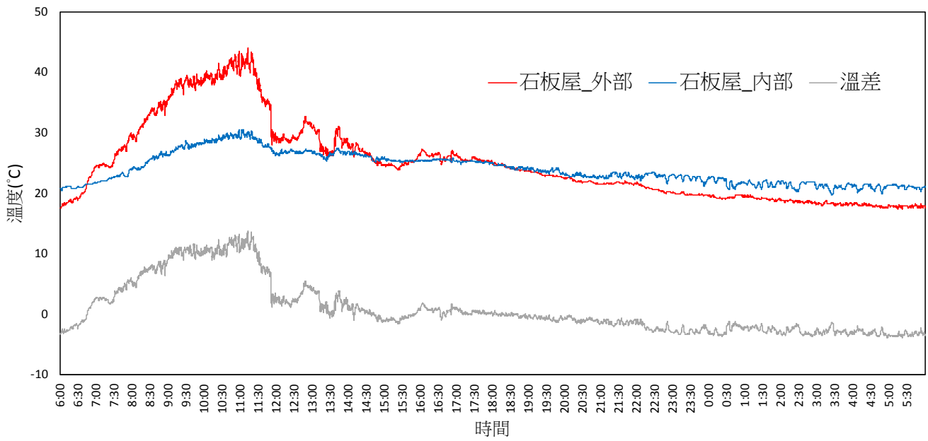
圖 9 真實環境中石板屋內外部溫度變化情形
