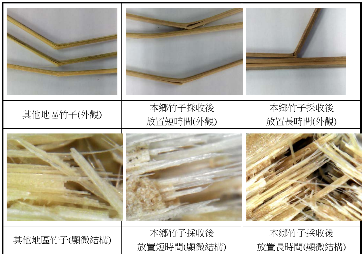
圖 4 竹子抗彎試驗斷裂情形
